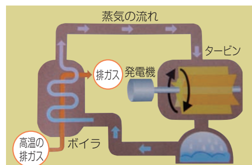
ボイラ・タービンのしくみ
